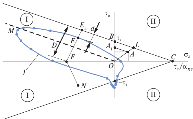
Рис. 1. Диаграмма Данг Вана циклической усталости при многоосном нагружении:
