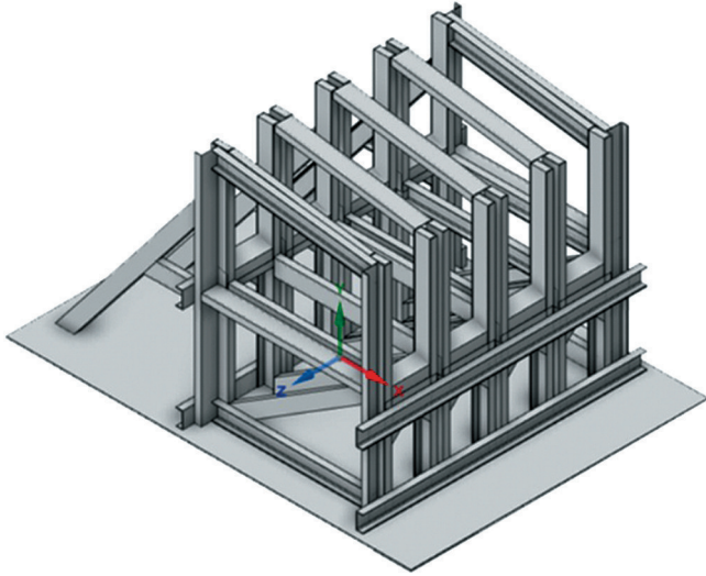
Рис. 2. Предлагаемое удерживающее устройство для длинномерного груза*
