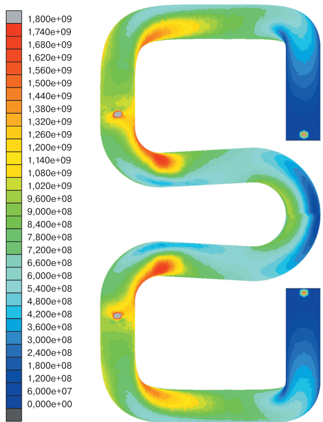
Рис. 4. Напряженно-деформированное состояние упругой клеммы Skl 14 при виртуальном прогибе центральной петли*
