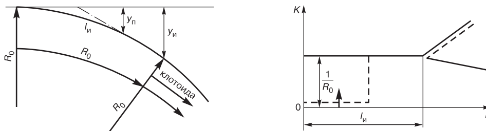
Рис. 3. Геометрические схемы острых (слева) и кривизна стрелочных кривых в зоне острых (справа) в виде комбинации клотоида и круговой кривой с увеличением кривизны, или с уменьшением кривизны*
